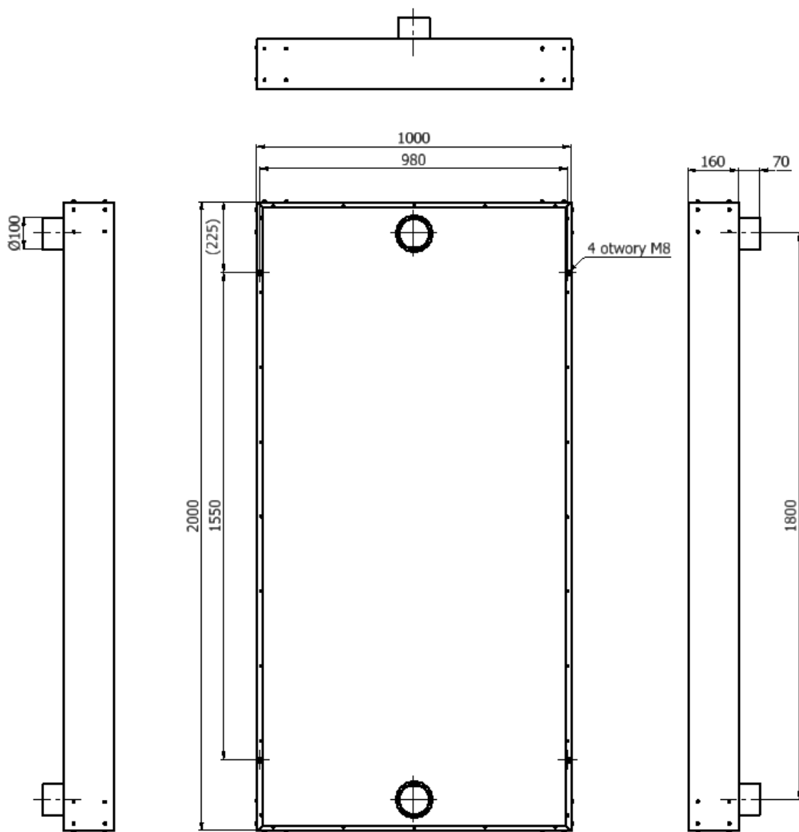
Rys. 1 Wymiary gabarytowe i rozstaw otworów montażowych kolektora.
